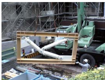
トグル装置の吊り上げ
