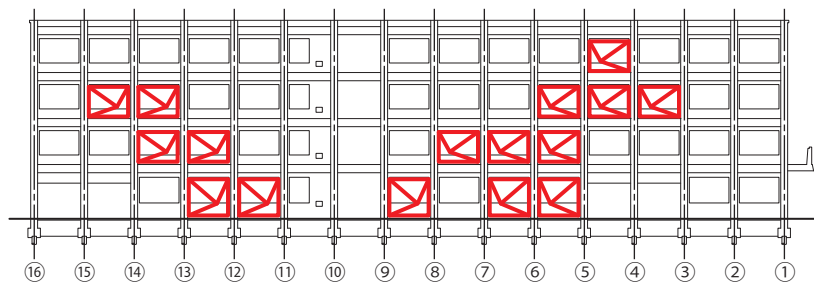
北側軸組図 (A 通り)
