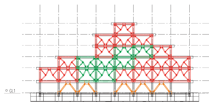
南側構造図
